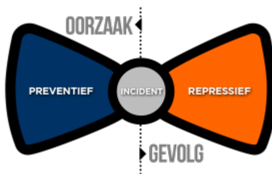
Figuur 15: Vlinderdasmodel
